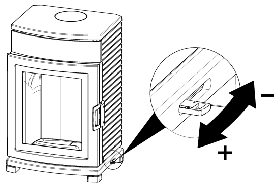
Fig. 4: Luftschieber regulieren
